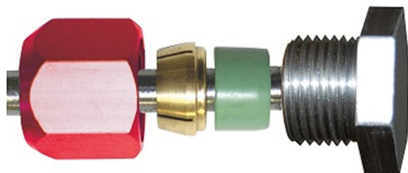
57. 007935020700 Korek 12mm OD
